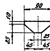
Разрез по 1-1
